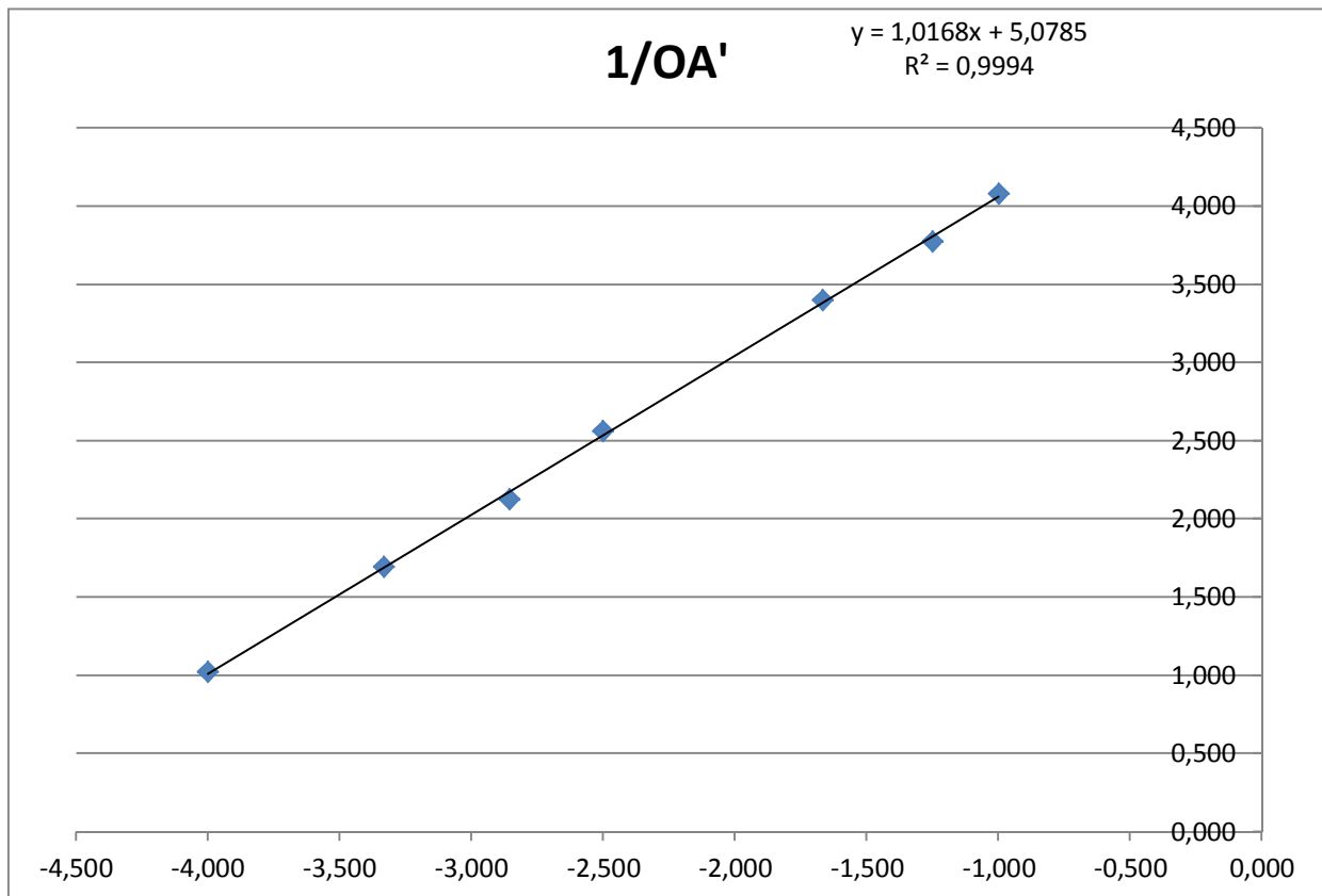
Relation de conjugaison pour une lentille mince convergente
